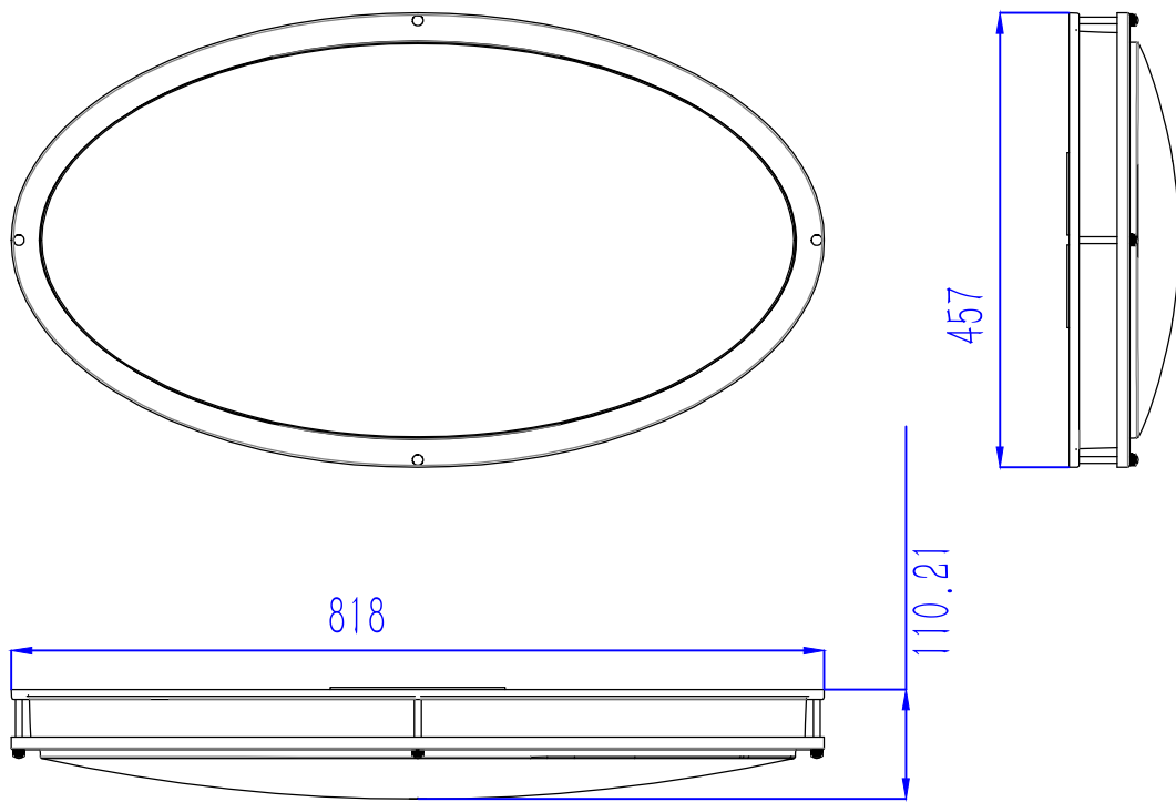
A32吸顶灯
