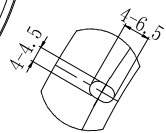
部详图 4:1
