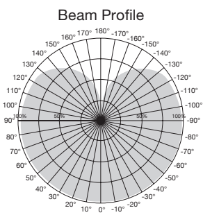
Beam Angle: 280°
